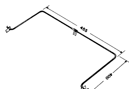
1214 950W Oven Element Replaces - Chef 02519
