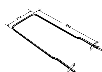
1228 1500W Rotisserie Element Replaces - Chef 02557
